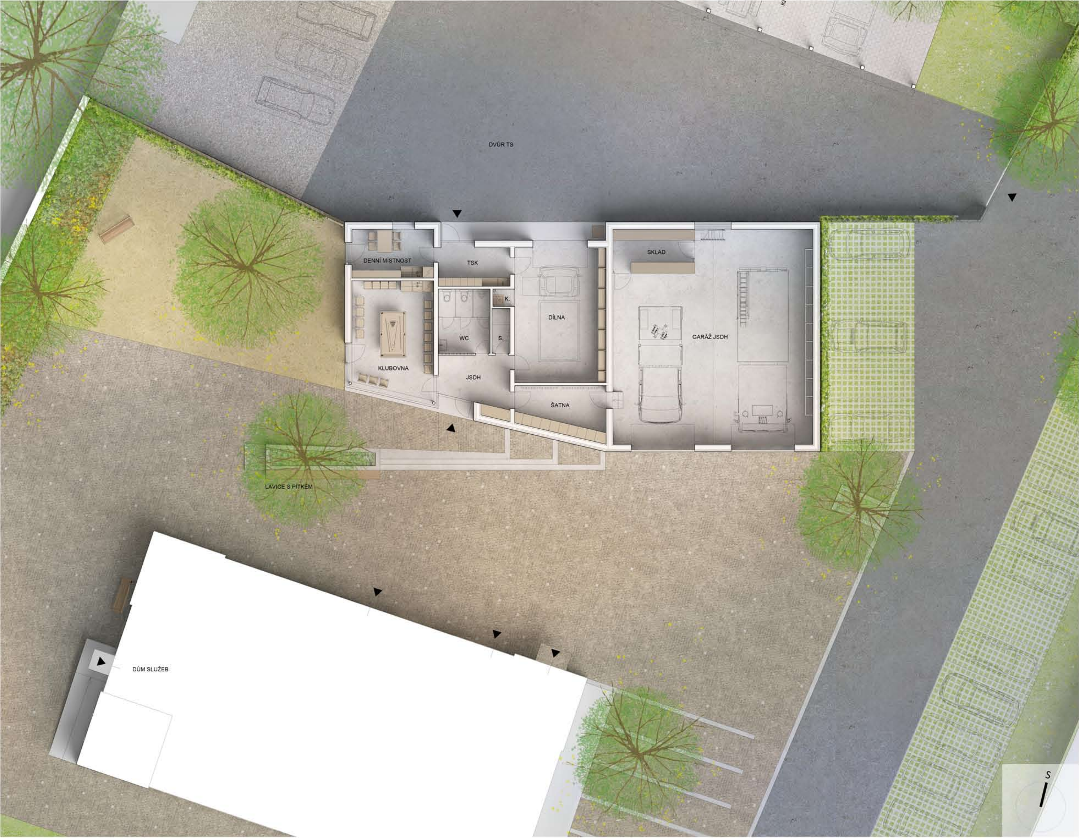
PŮDORYS HLAVNÍHO OBJEKTU M 1:100
