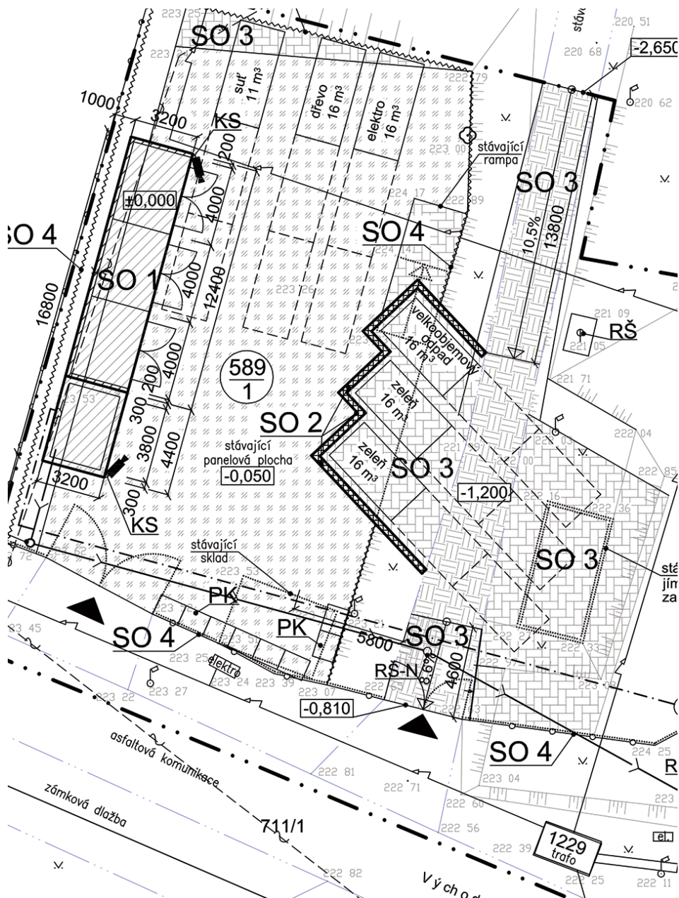
-IČ- Návrh uspořádání kontejnerů
